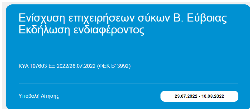
Εικόνα 2. Οθόνη εφαρμογών
