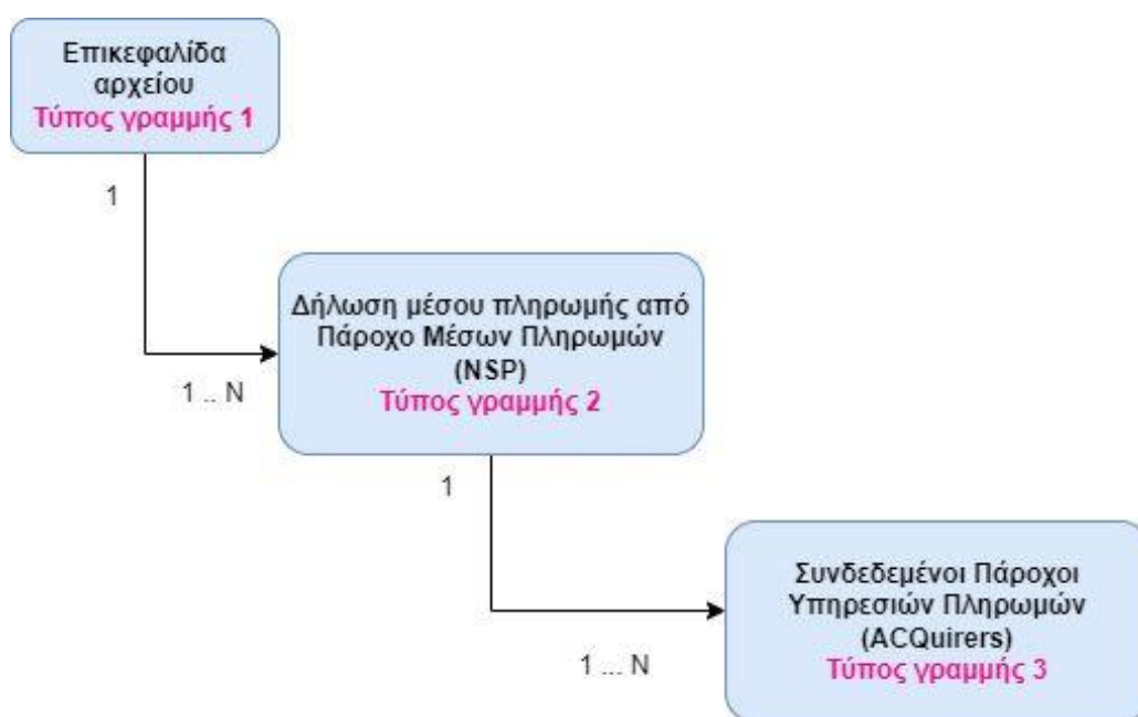
Εικόνα 1. Ιεραρχία αρχείου CSV για NSPs
