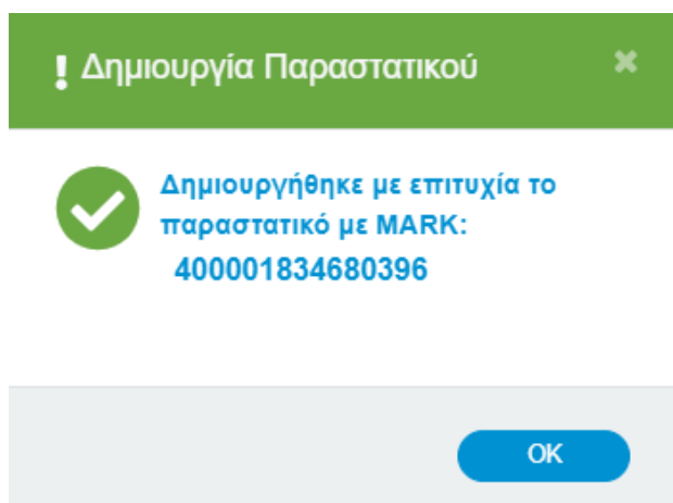
Εικόνα 35. Δημιουργία MARK
