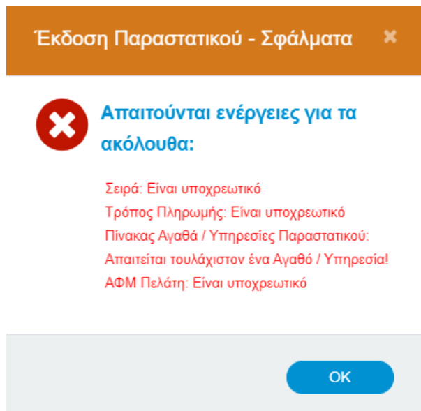
Εικόνα 13. Παράθυρο σφαλμάτων
