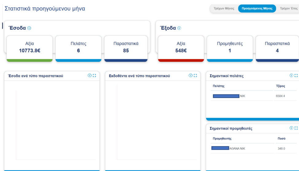
Εικόνα 39. Στατιστικά
