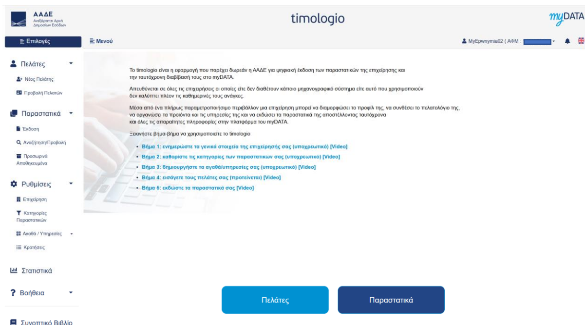
Εικόνα 5. Εισαγωγική οθόνη
